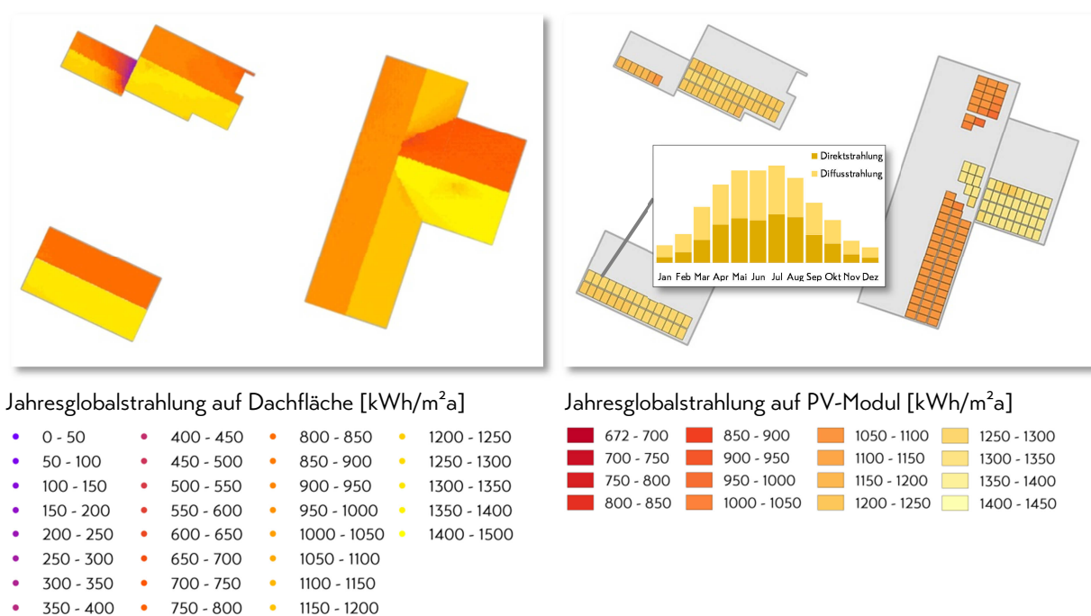
Abbildung 16: Simulation der solaren Einstrahlung auf Dachflächen (links) und Ergebnis der technischen Potenzialanalyse für Photovoltaikmodule mit monatlicher Auflösung von Direkt- und Diffusstrahlung (rechts)
