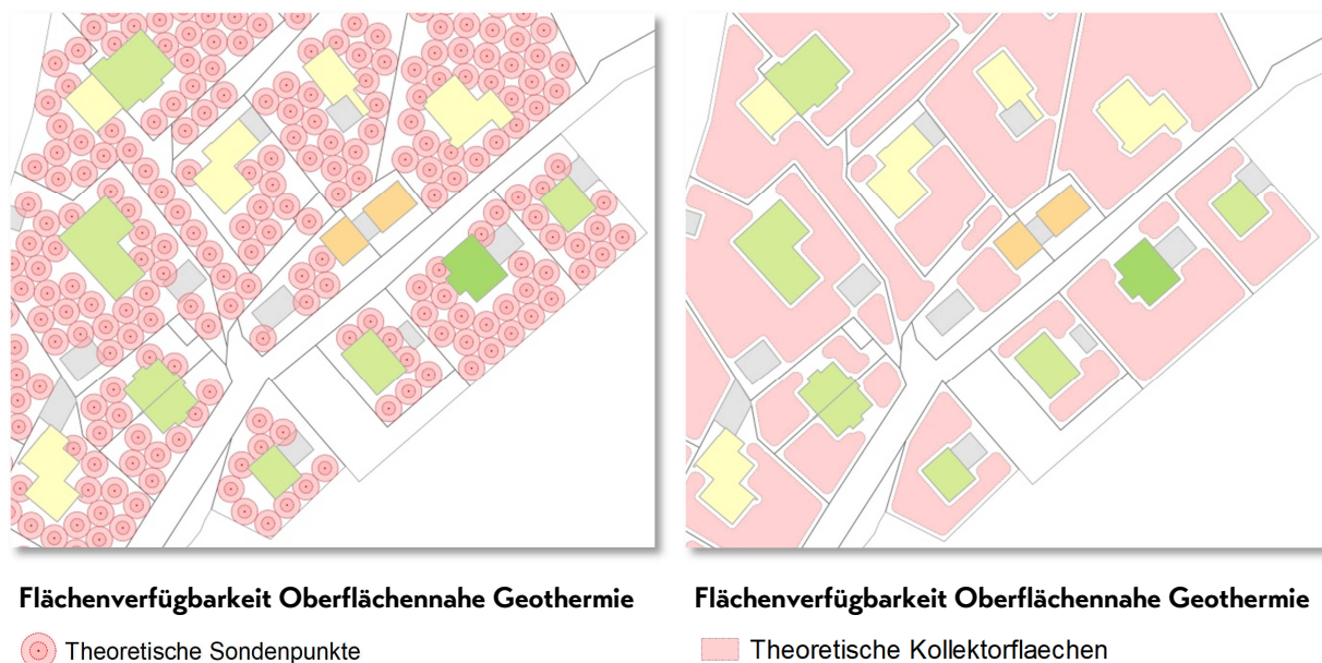
Abbildung 20: Beispielhafte Darstellung der Analyseergebnisse zur theoretischen Flächenverfügbarkeit für Erdwärmesonden und Erdwärmekollektoren
