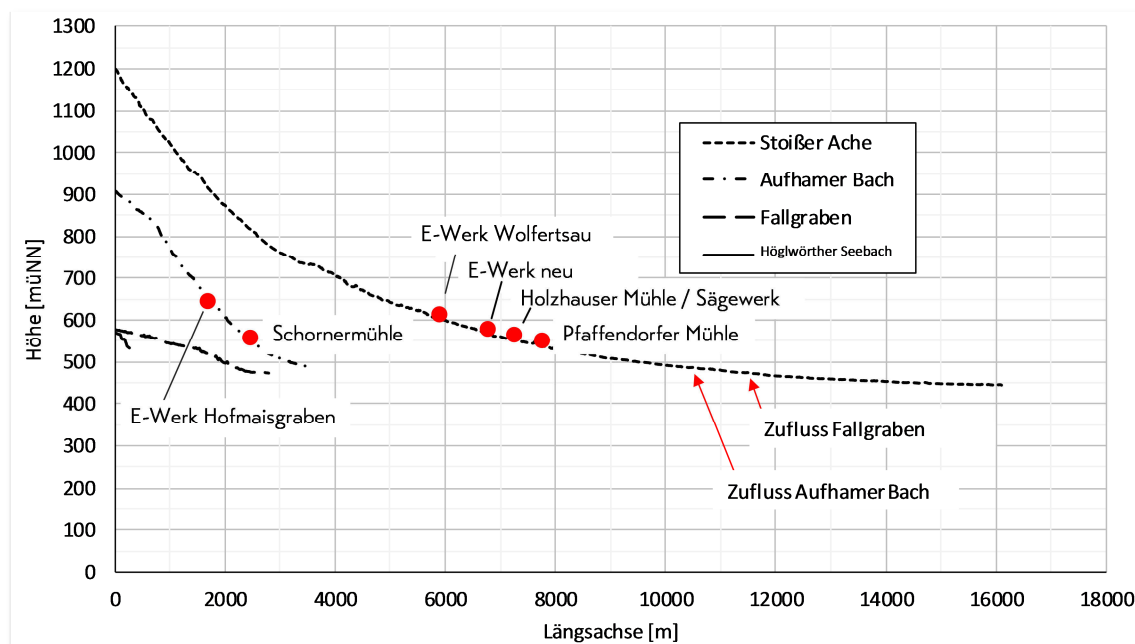
Abbildung 35: Höhenprofil Stoßer Ache
