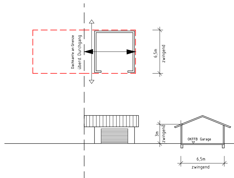
FALL 2: einseitiger Grenzanbau mit Durchgang
