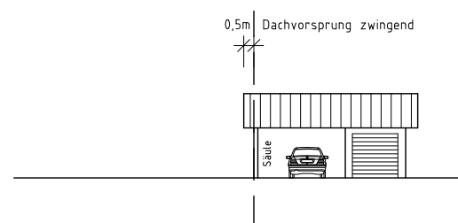
FALL 3: einseitiger Grenzanbau mit Carport + Durchgang
