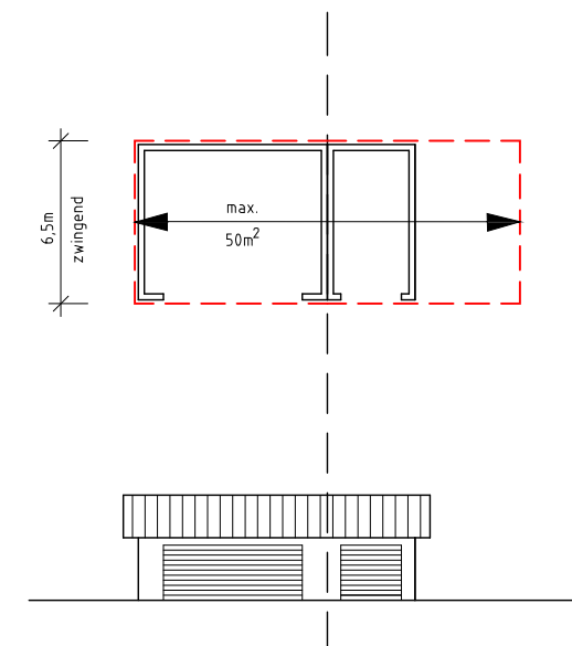
FALL 5: zweiseitiger Grenzanbau ohne Durchgang (ungleiche Garagengröße)
