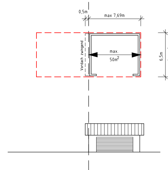
FALL 5: zweiseitiger Grenzanbau ohne Durchgang (ungleiche Garagengröße)
