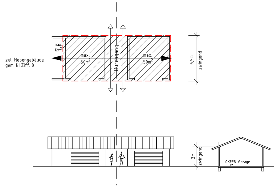
FALL 1: doppelseitiger Grenzanbau mit Durchgang
